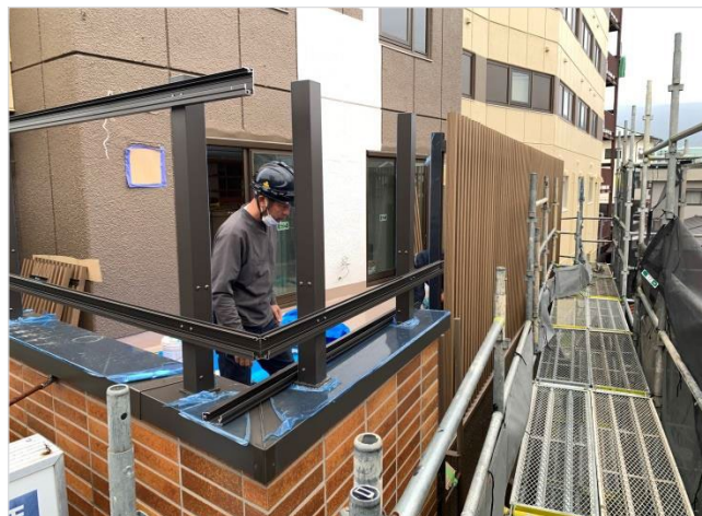
[工事種別] 鋼製建具工事 [作業内容] 2Fフェンス設置
